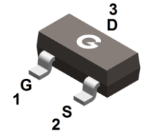
BL3407-3L SOT-23-3L
